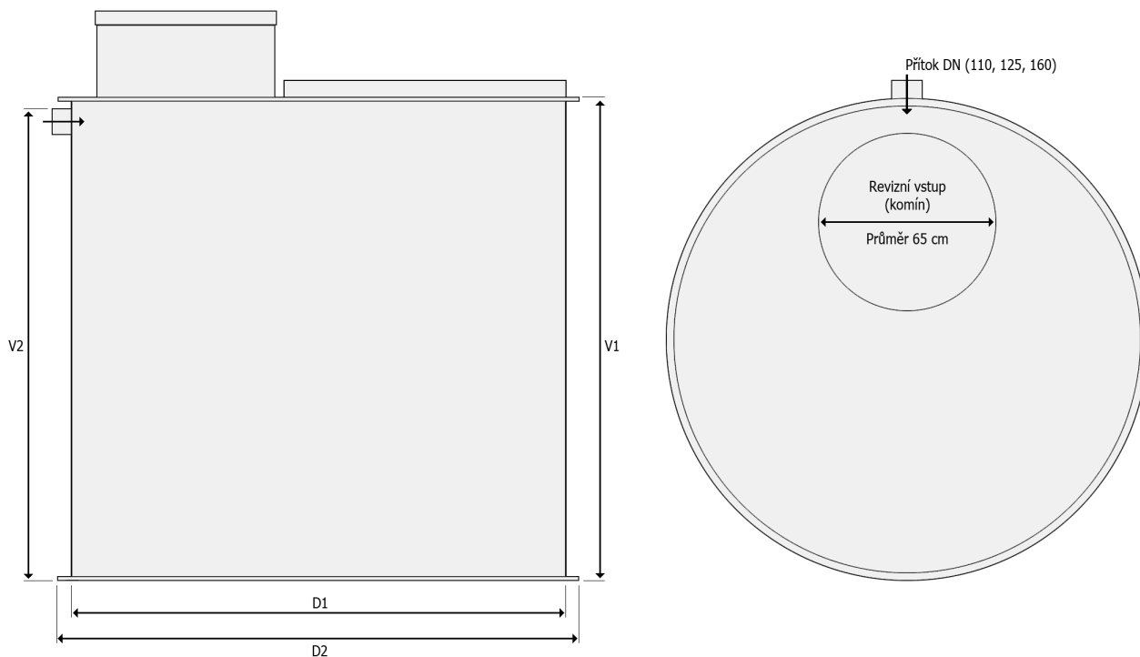
PLASTOVÉ JÍMKY - ŽUMPY, NA ODPADNÍ VODU, VÁLCOVÉ - K OBETONOVÁNÍ (standardní rozměry)
