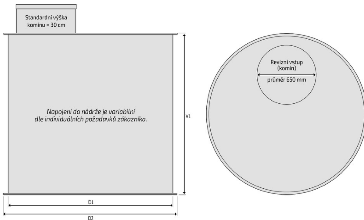
PLASTOVÉ NÁDRŽE - NA PITNOU VODU, VÁLCOVÉ - K OBETONOVÁNÍ (standardní rozměry)
